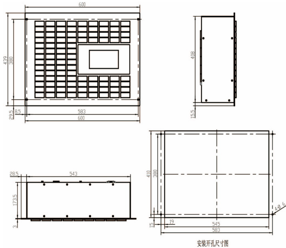
图 3 FYXH-96YJ-A 外形尺寸及安装图
