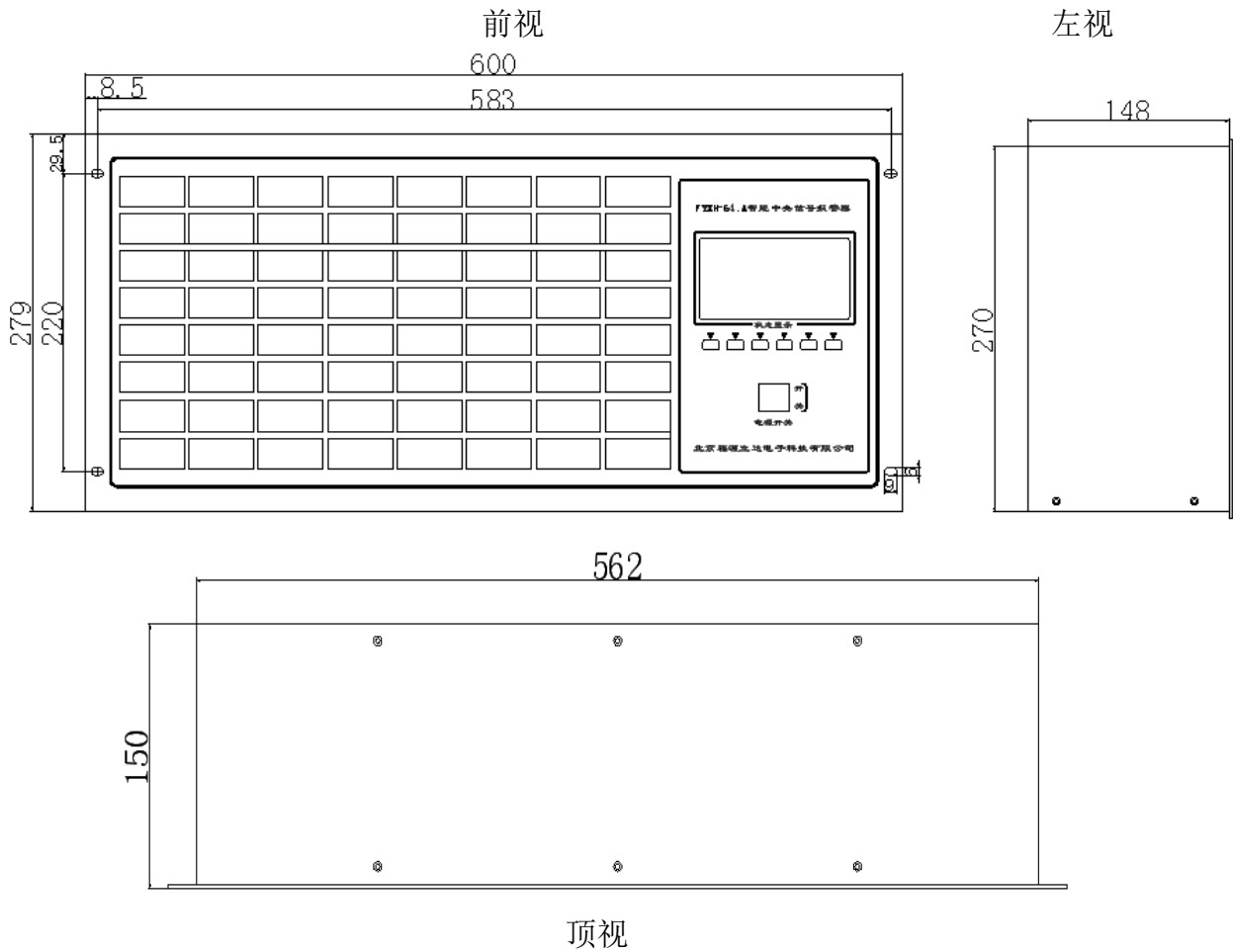
FYXH-64YJ-B 外形尺寸图
