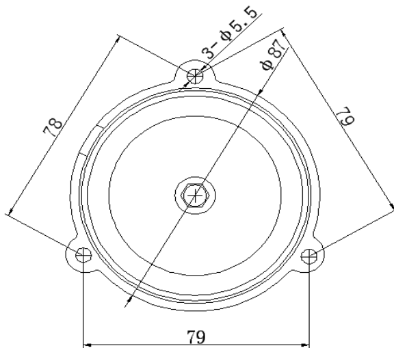
电铃的尺寸
