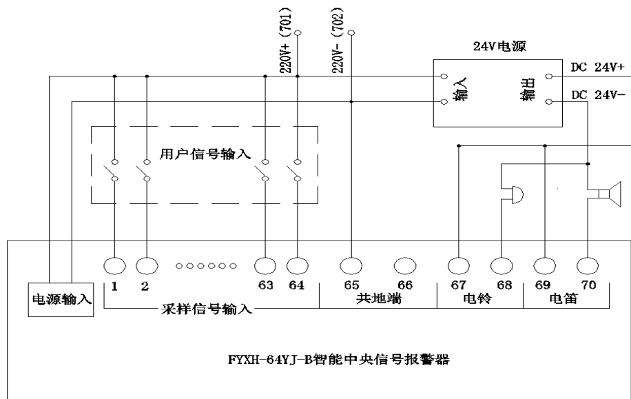
FYXH-64YJ-B 智能中央信号报警器接线图
