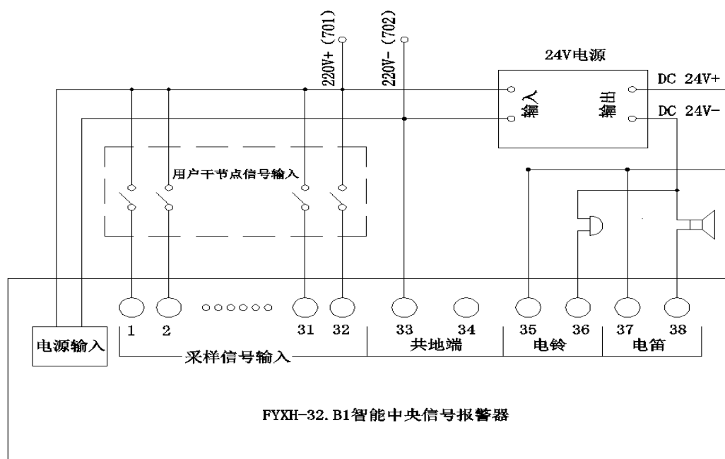
FYXH-32.B1 型智能中央信号报警器接线原理图
