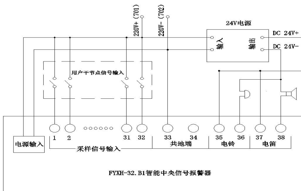
FYPH-32. B1 型智能中央信号报警器接线原理图
