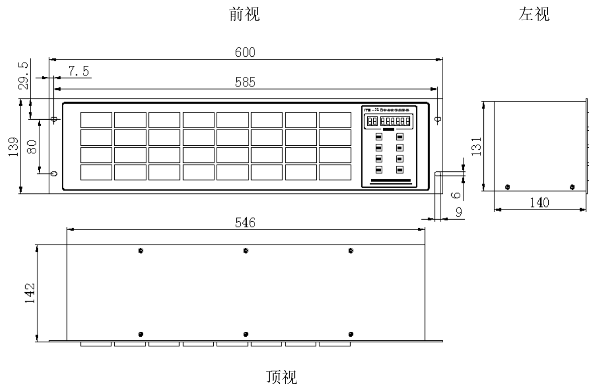
FYXH-32. B1 外形尺寸图
