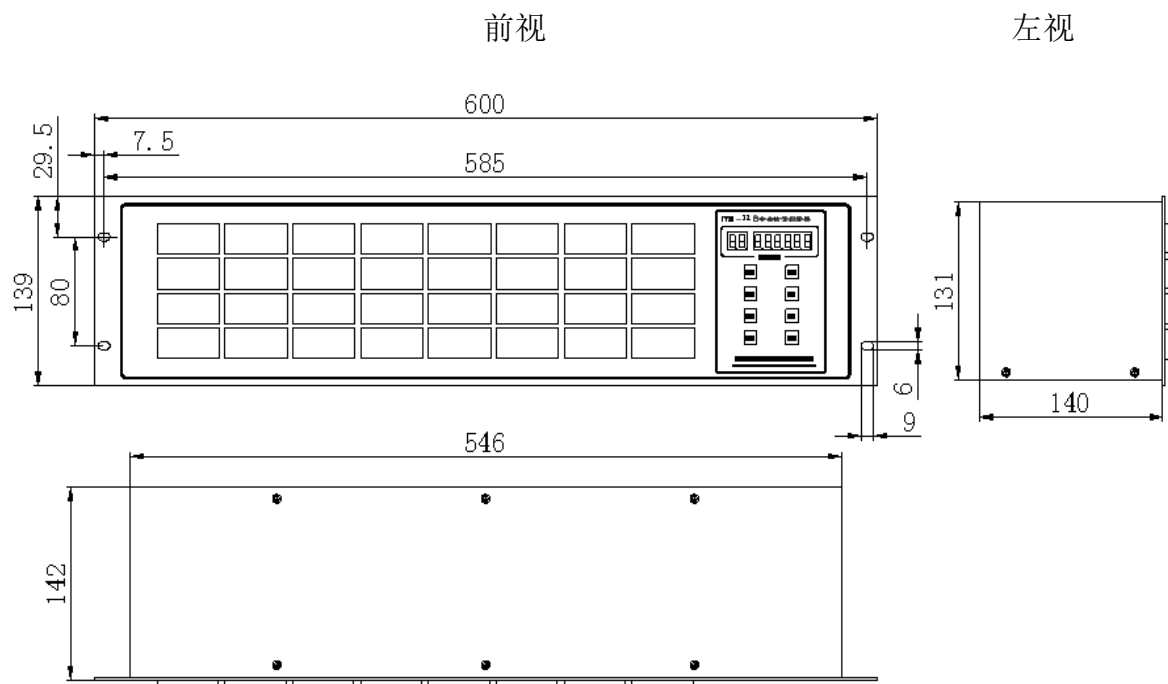
顶视 FYXH-32. B1 外形尺寸图
