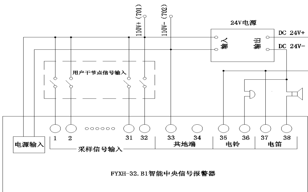
FYXH-32. B1 智能中央信号报警器接线原理图
